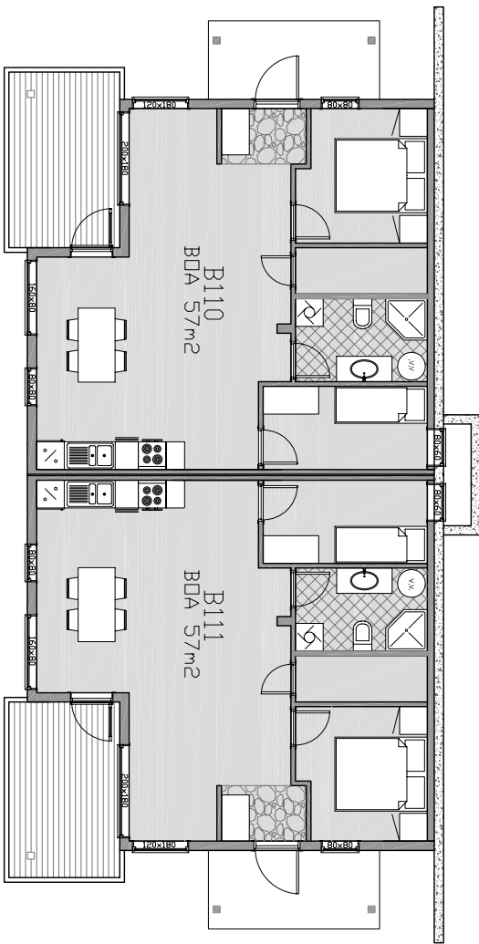
Bygg B3 1Etg.
